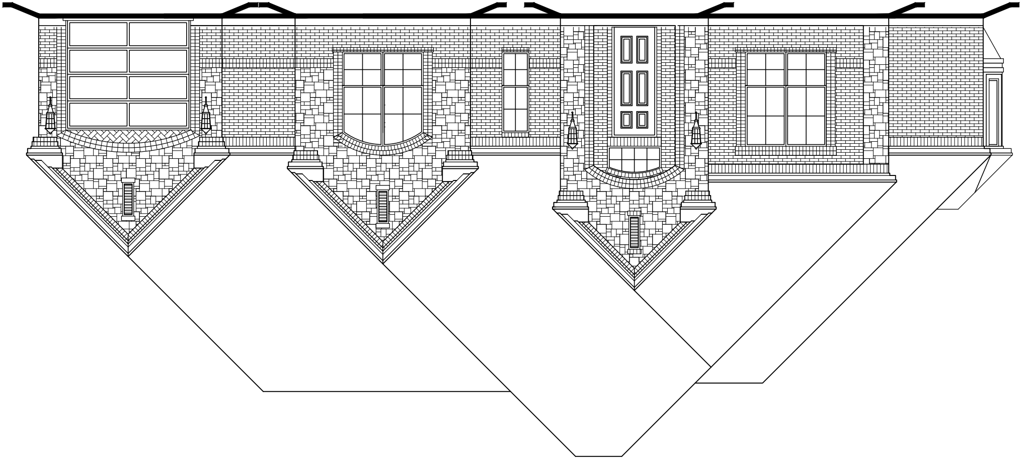
Elevation - A
