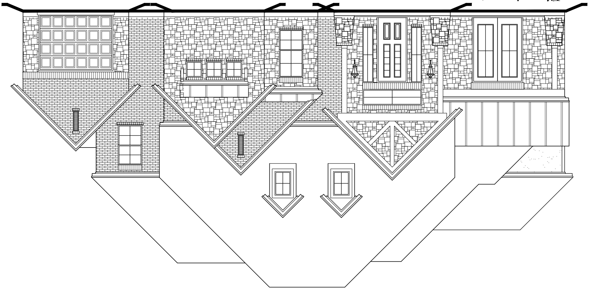
Elevation - A
